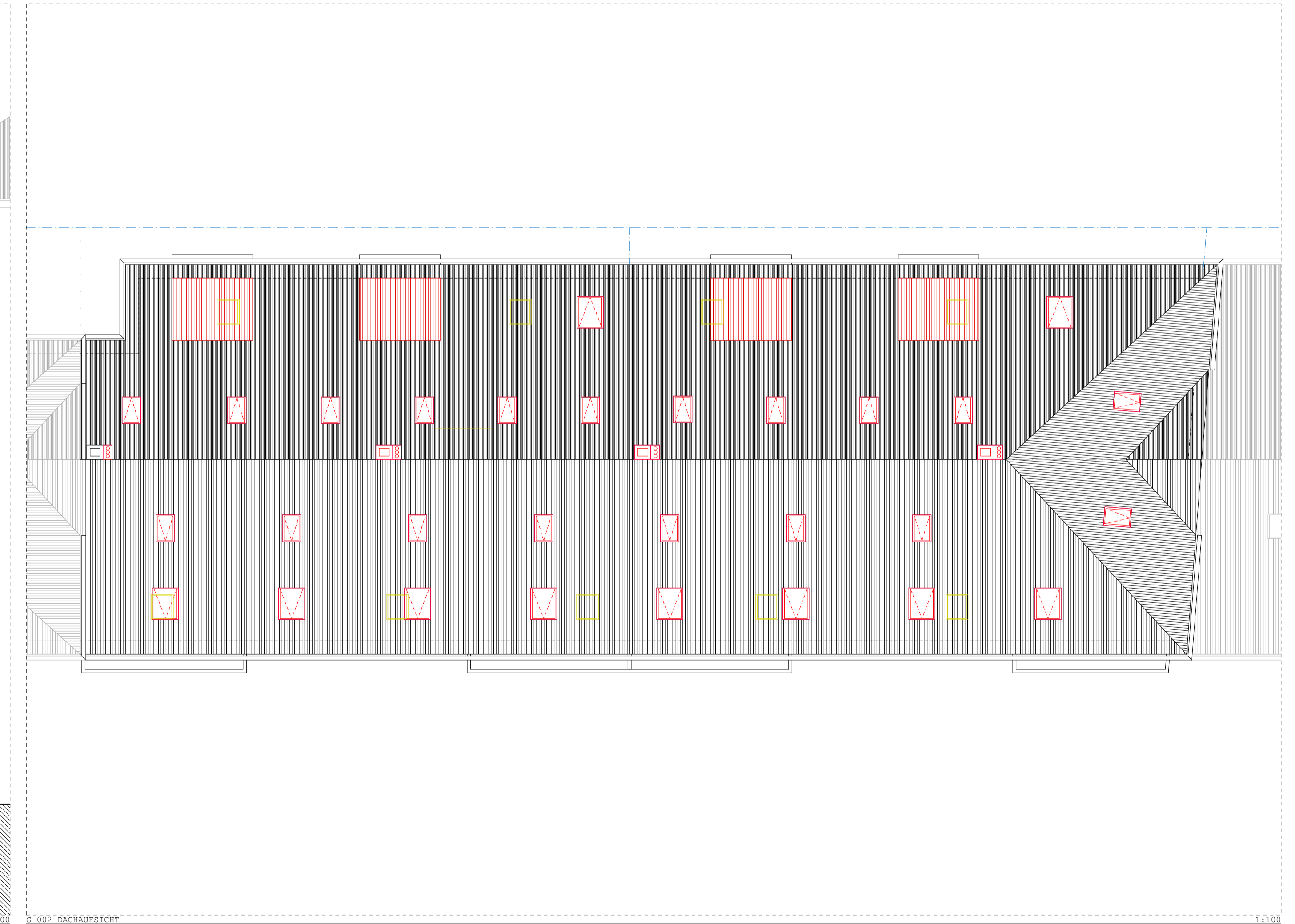
B_002 DACHANSICHT 1:100
